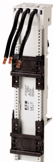
Busbar adapter, 55 mm, 63 A, DIN rail: 2
